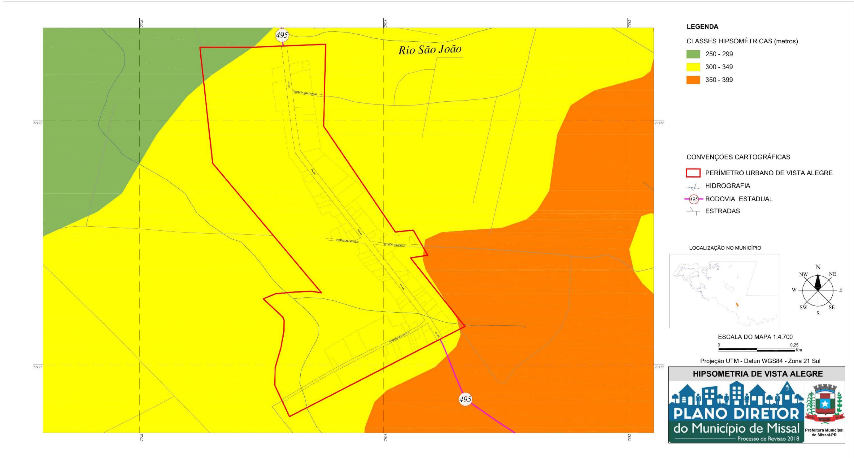
Mapa 11: Hipsometria do Núcleo Urbano de Vista Alegre
